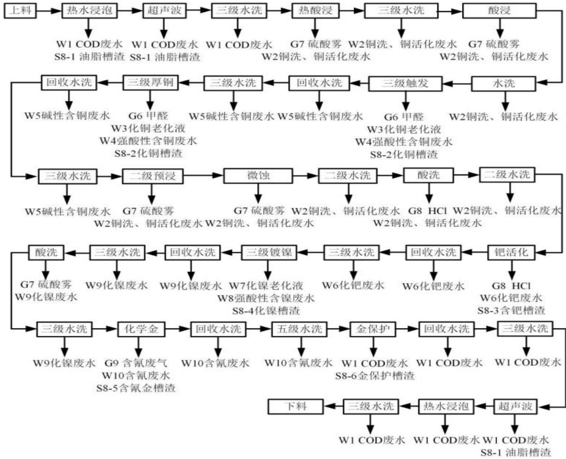
图 4.3.1-5 NPI 流程图
