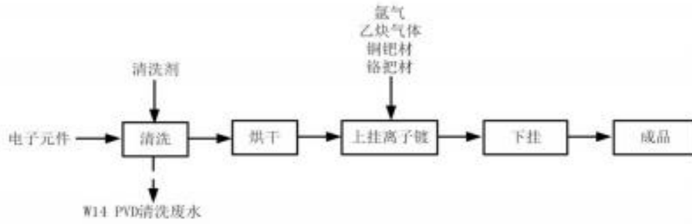
图 4.3.1-2 PVD 生产线
