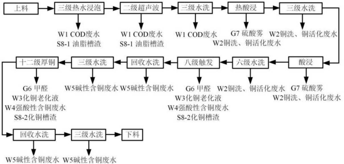
图 4.3.1-8 化学镀铜流程图
