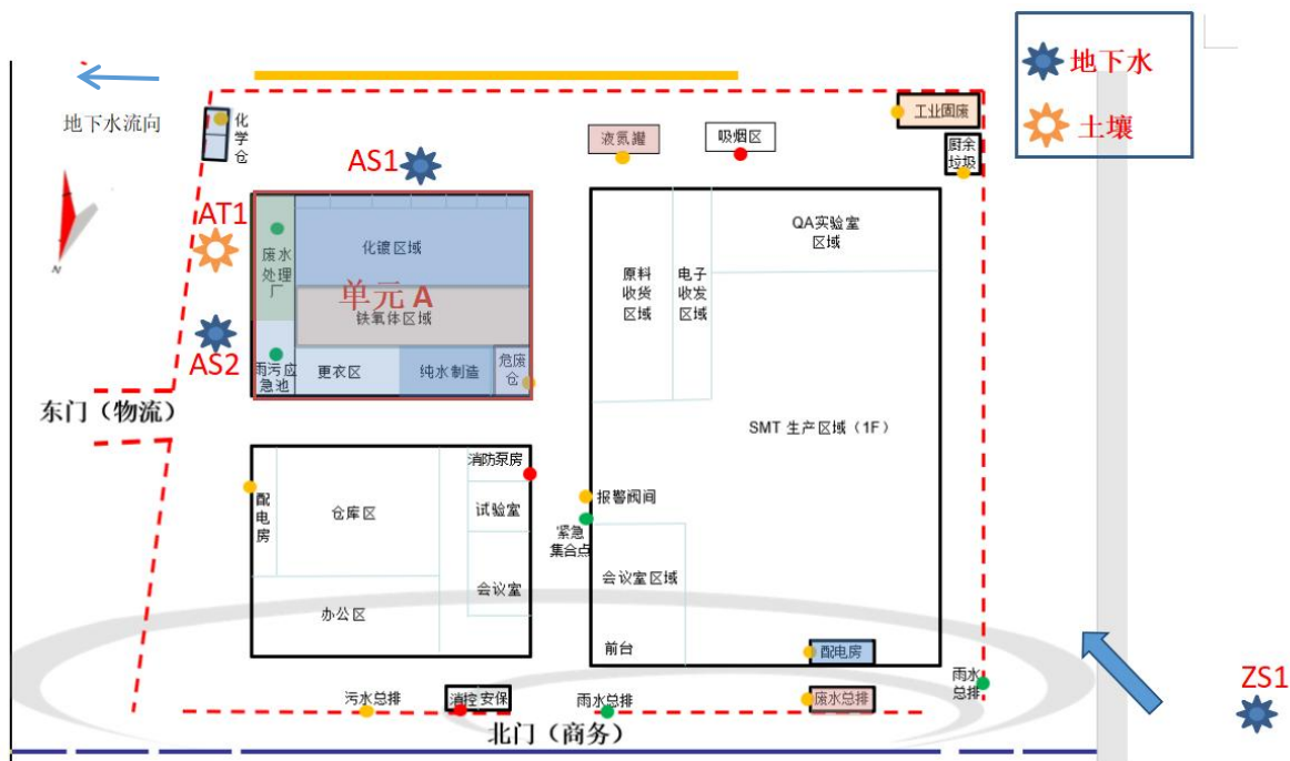
图 6.1-1 点位布置图
